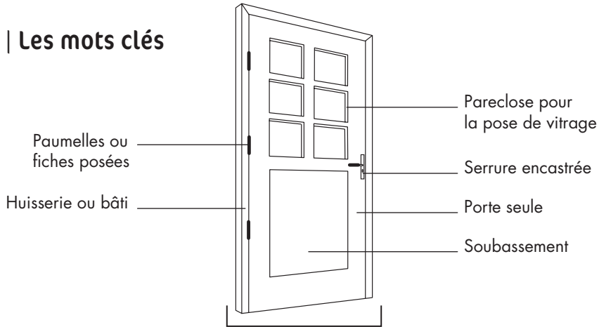
Bloc Porte (bâti + porte)
